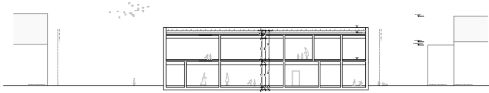
Schnitt A-A
